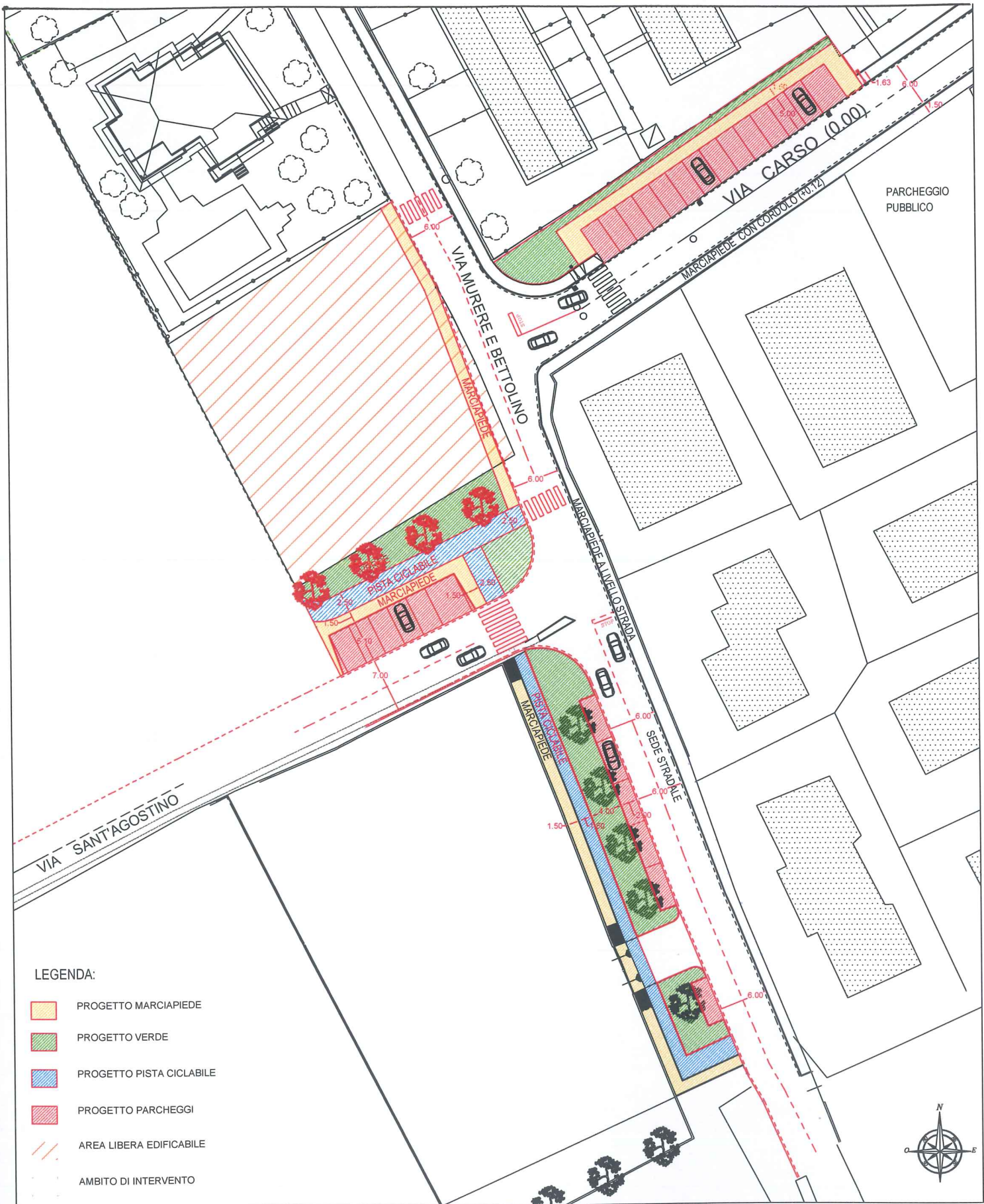
ALLEGATO B - RETTIFICA ASSETTO VIABILISTICO - VIE SANT'AGOSTINO / MURERE E BETTOLINO / CARSO
